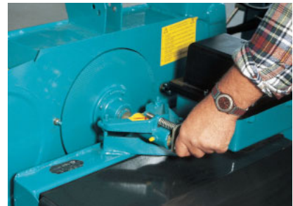
Messerschleifapparat zum schnellen Nachschleifen Knife grinding attachment for quick regrinding
