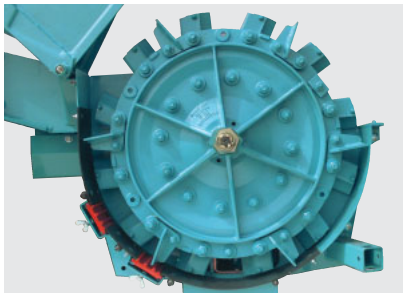
Messerscheibe mit Riffelplatte + Verschleißblech Knife rotor with shredder plate and wearing plate
